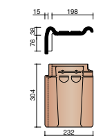
P044 7380 ● Tuile de rive à bord recourbé gauche
