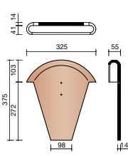
P000 1241 Fronton 230 mm "grande hauteur" NOUVEAU
