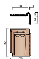
P044 7390 ● Tuile de rive à bord recourbé droite
