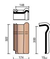
P044 8530 ☼ ● 3/4 tuile faîtière
