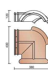
P000 5120 Rencontre 2 faîtières 230 mm et 1 arêtier 190 mm
