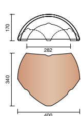
P000 5500 Jonction 1 faîtière 230 mm et 2 arêtiers 230 mm
