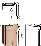
P044 8875 ☼ Pièce d'angle pour tuile faîtière
