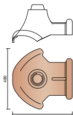
P000 5290 Rencontre porte-boule 1 faîtière 230 mm et 2 arêtiers 190 mm (+ 5900 ou 5950 )
