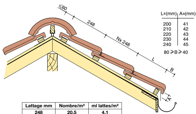
COTATIONS SUR RAMPANT
