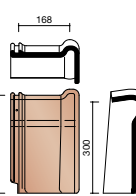
P044 7590 ● Tuile faîtière de rive droite
