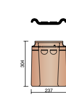
P044 8350 ☼ ● Tuile à bord recourbé et double bourrelet
