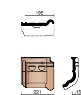
P044 8200 ● Tuile membron (5,2 au ml)
