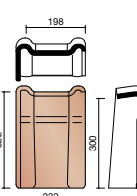
P044 7580 ● Tuile faîtière de rive gauche
