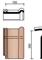
P044 8500 ● Tuile faîtière (5,2 au ml)
