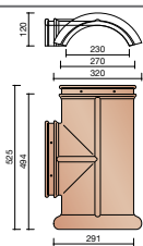
P000 5020 Rencontre 3 faîtières 230 mm
