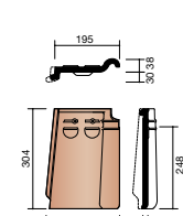
P044 8870 ☼ Pièce d'angle
