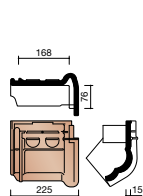
P044 7290 ● Tuile membron de rive droite
