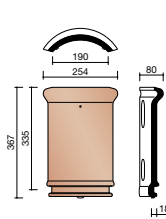
P000 3100 Arêtier demi-rond 190 mm (3,0 au ml)
