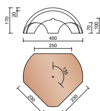
P000 5740 Jonction 1 faîtière 230 mm et 2 arêtiers 190 mm
