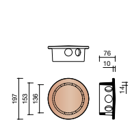
P000 8750 Mitron d'aération Ø 100 mm
