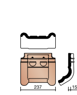
P044 8250 ☼ ● Tuile membron à double bourrelet
