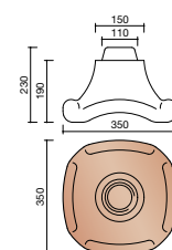
P000 5640 Rencontre 4 arêtiers 190 mm avec porte-boule (+ 5900 ou 5950 )
