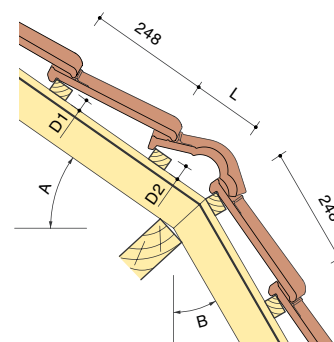
POSE MEMBRONS POUR RACCORDS TOITURE / FAÇADE
