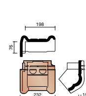
P044 7280 ● Tuile membron de rive gauche
