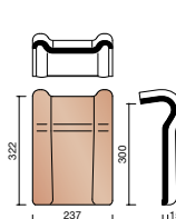
P044 8550 ☼ ● Tuile faîtière à double bourrelet
