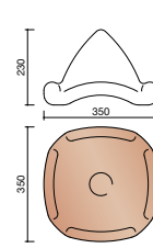
P000 5630 Rencontre 4 arêtiers 190 mm sans porte-boule
