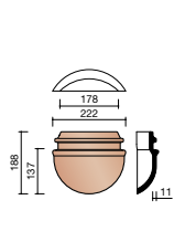
P000 3110 About d'arêtier demi-rond à emboîtement 190 mm
