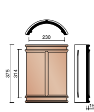
P000 1230 Faîtière demi-ronde à double emboîtement 230 mm
