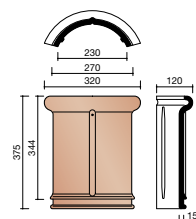
P000 1200 Faîtière demi-ronde 230 mm (3,0 au ml)
