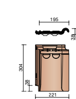
P044 8610 Tuile chatière (12 cm²) (0,17 pc / m² projeté) ♦
