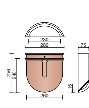
P000 1260 About d'arêtier demi-rond à emboîtement 230 mm
